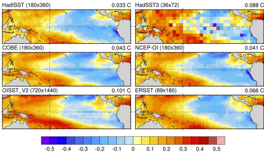
Trend (degC/decade) : 1982-2010
