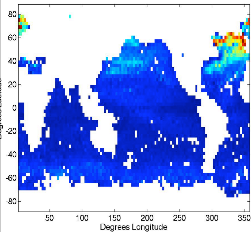
ARGO MLD JFM
