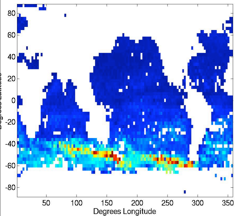
ARGO MLD JAS
