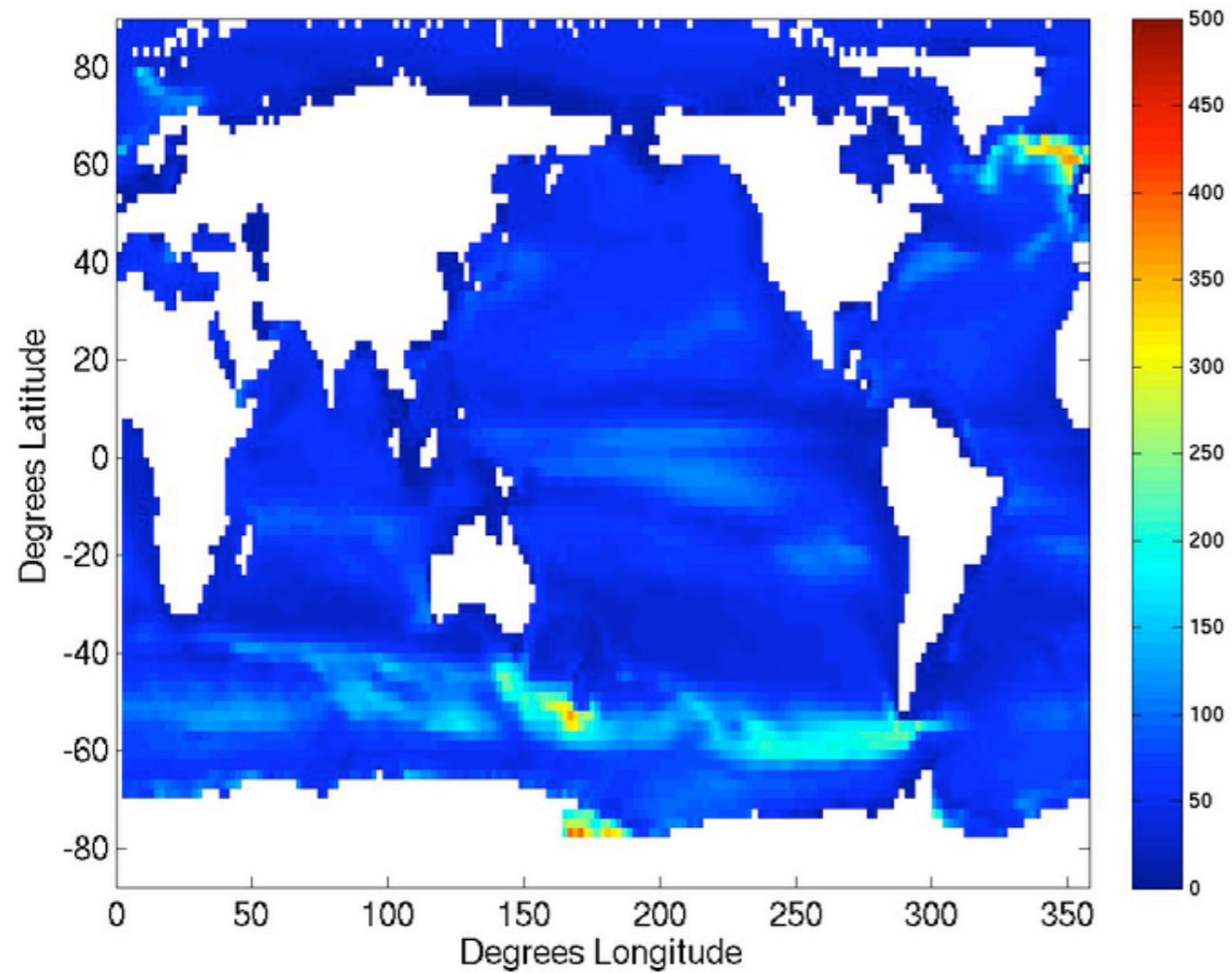
CCSM Control MLD OND
