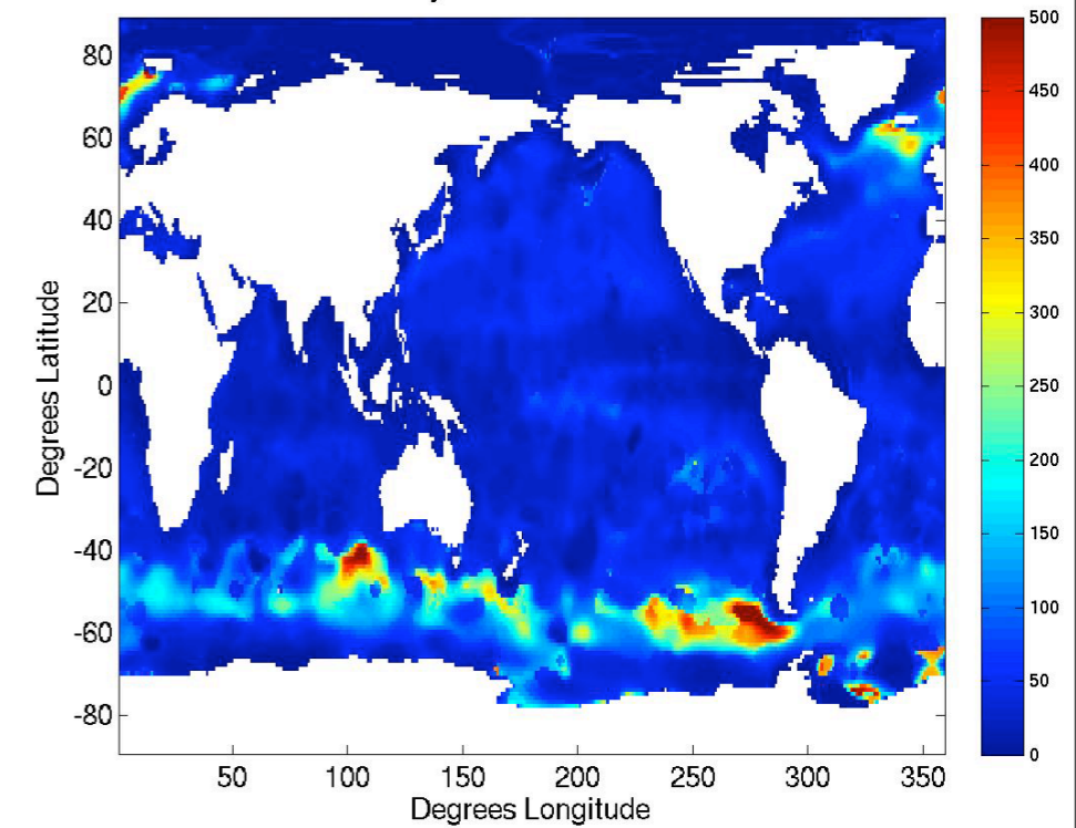
Monterey and Levitus MLD OND
