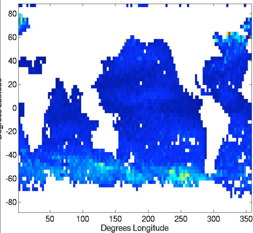
ARGO MLD AMJ
