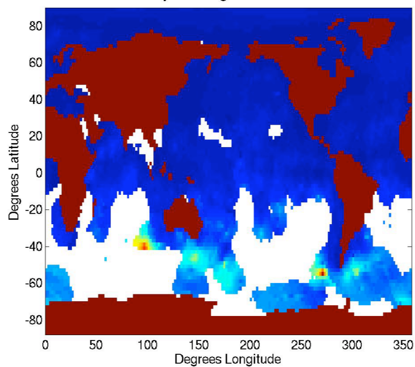
de Boyer-Montegut et al. MLD JAS
