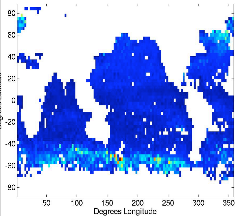
ARGO MLD OND
