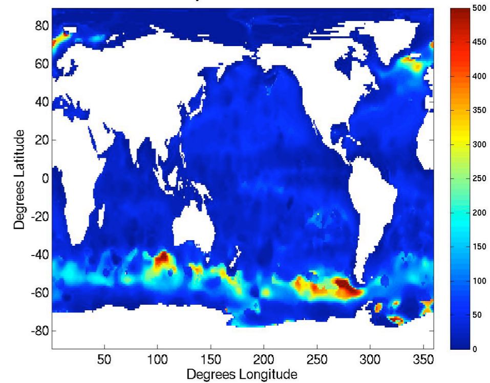
Monterey and Levitus MLD OND
