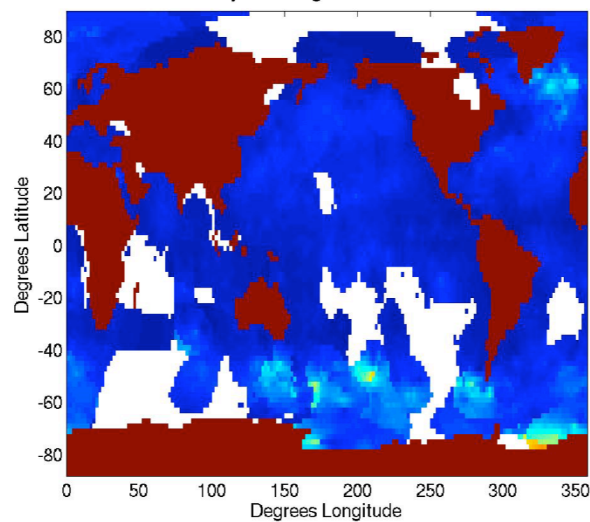
de Boyer-Montegut et al. MLD OND
