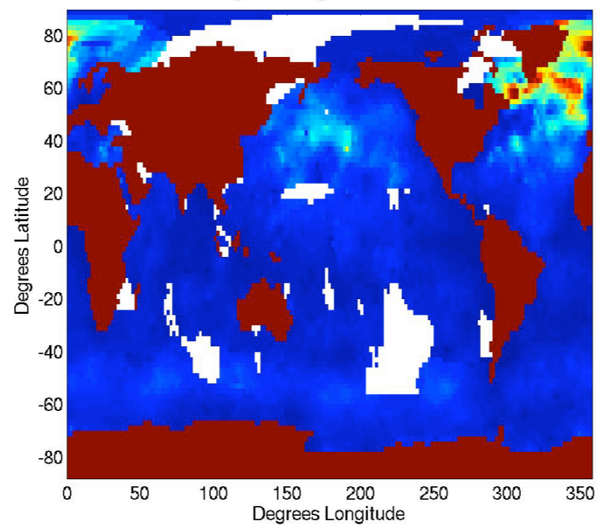
de Boyer-Montegut et al. MLD JFM
